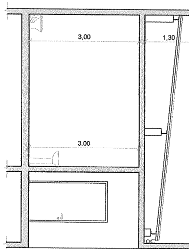
CORTE CC
