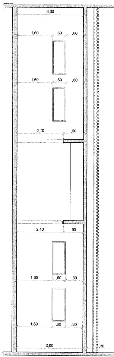
CORTE BB
